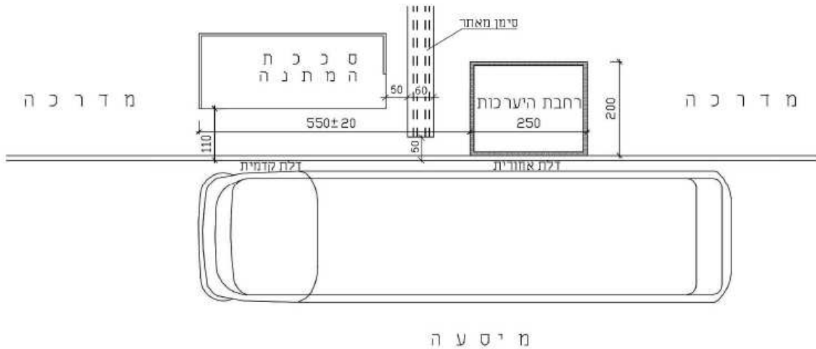
20 א – תחנת אוטובוס עם סככת המתנה
