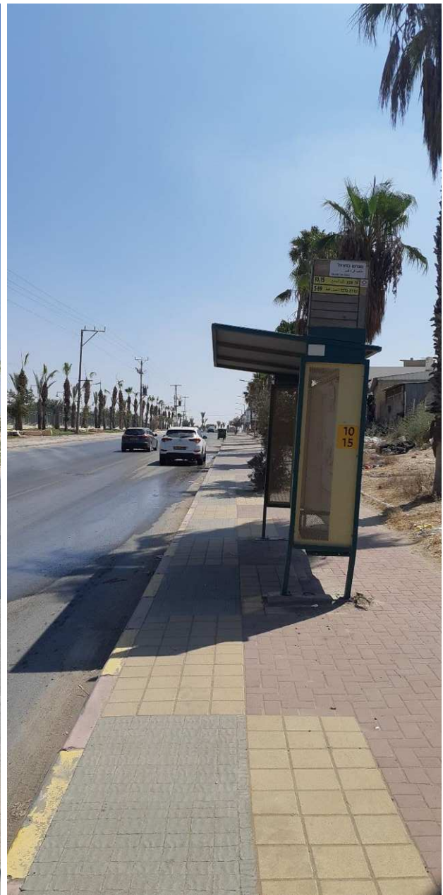
יש לרצף את המדרכה בצבע אחיד , מכיוון שריבוי צבעים מפריע לאנשים בעלי מוגבלות בראייה ולא מאפשר להם לזהות את המדרכה התחנה ומקשה על התמצאות במרחב
