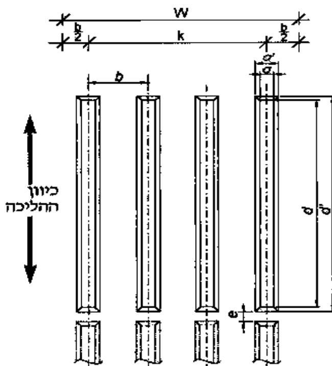
25 - מבט על
