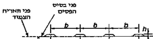
26 - חתך אנכי
